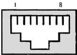
插座前视图
